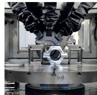
Endkonturfräsen am Zusammenbau © SLV Halle GmbH
