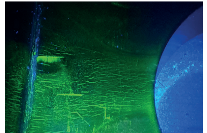
MT-Prüfung an einer gebrauchten Aluminiumdruckgussform im Bereich eines Auswerfers © SLV Halle GmbH
