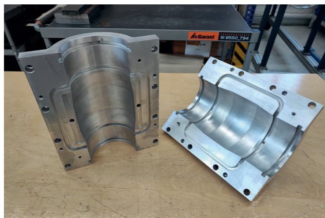
Endbearbeiteter Werkzeug-Prototyp © SLV Halle GmbH
