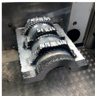
Additive Fertigung des Oberkastens © SLV Halle GmbH
