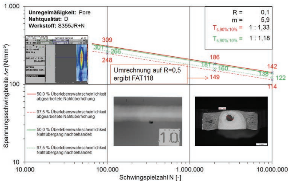
Wöhlerlinie - Bewertungsgruppe D – Pore – abgearbeitet (rot) und nachbehandelt (grün)
