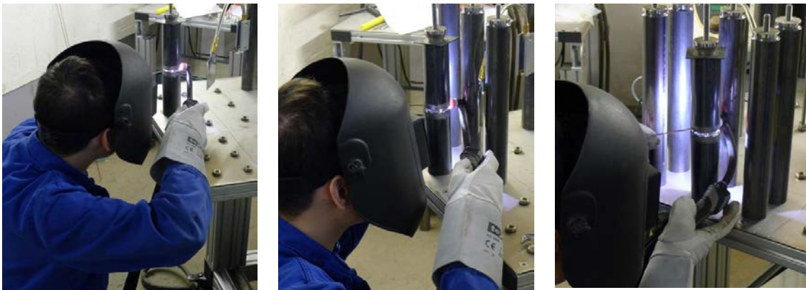
Schulung im Spiegelschweißen bei zunehmend eingeschränkter Zugänglichkeit
