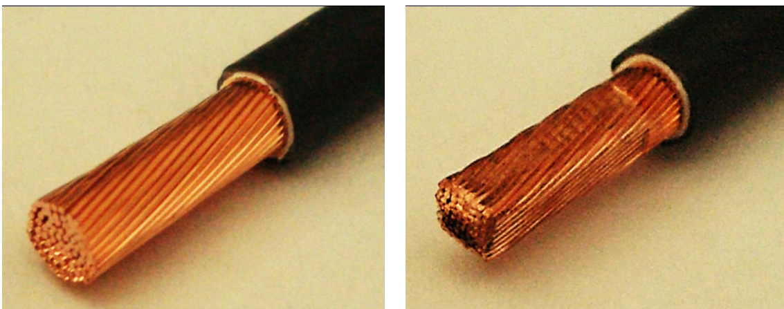
Links: Ausgangszustand; rechts: Widerstandskompaktierung einer 6 mm 2 -Kupferlitze
