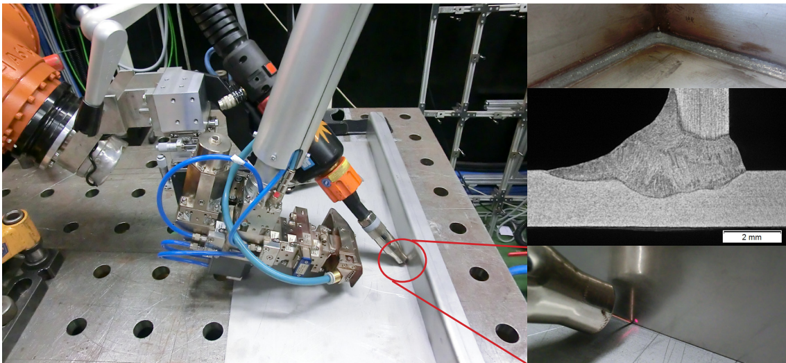
Technische Umsetzung des miniaturisierten Hybridschweißkopfes für eine Kehlnahtanwendung, eine beispielhafte Ausrichtung zum Schweißstoß und Beispiele für die Nahtausführung
