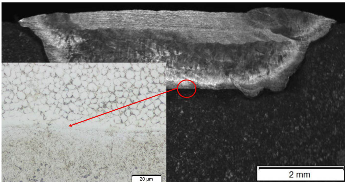
Querschnitt einer Laserstrahl-Reparaturschweißung mit Mikroaufnahme des Übergangs Schweißgut und Wärmeinflusszone am Substrat X20Cr13
