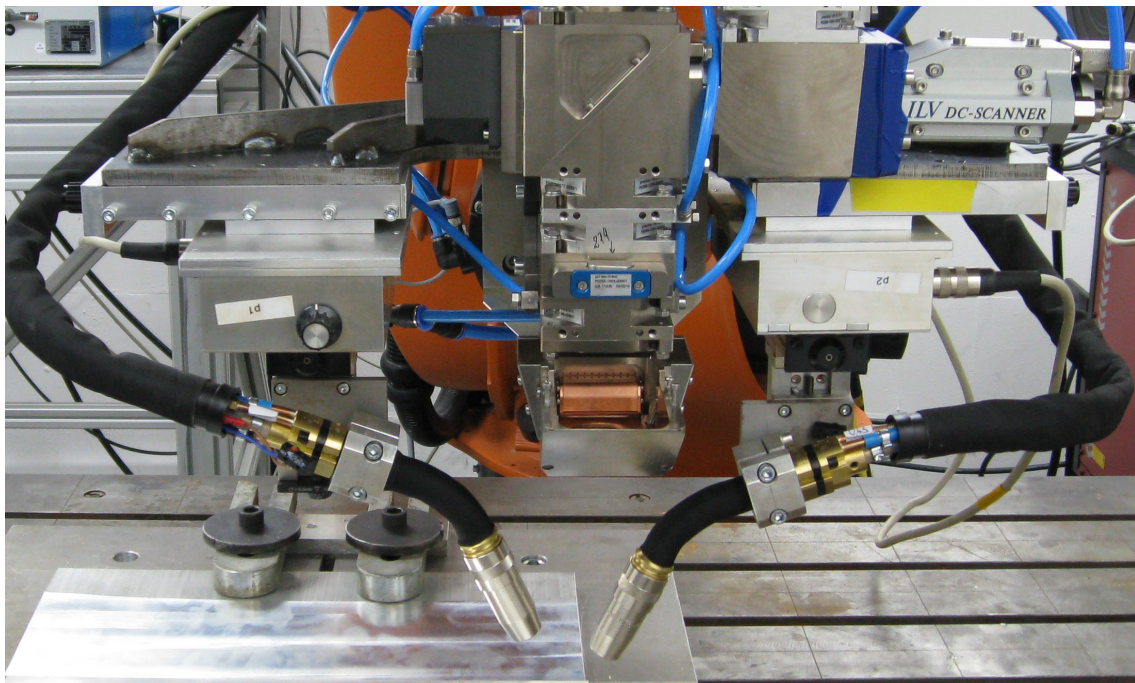
Arbeitskopf mit den integrierten Freiheitsgraden
