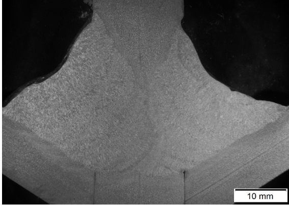
Makroschliffbild einer MSG-Reparaturschweißung mit Fülldraht
