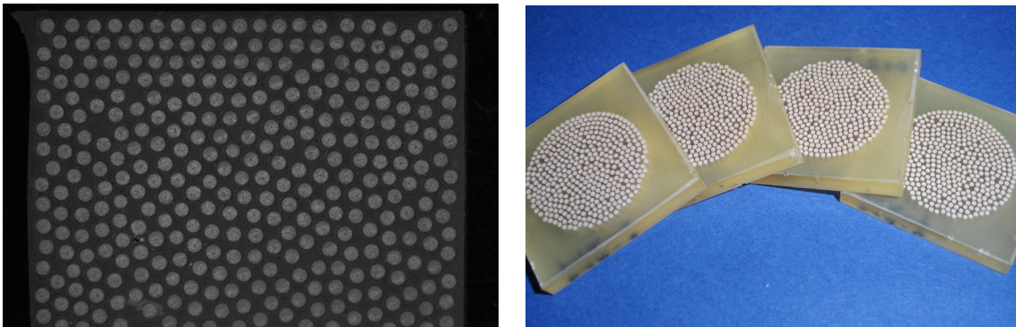
Links: Schliffbild eines Faserkomposits mit einem Fasergehalt von 40 %; rechts: Faserkompositscheiben vor dem Aufbringen der Elektroden
